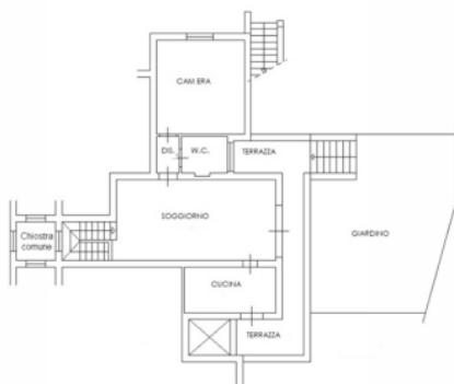
PIANO RIALZATO
